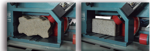
Acessório para fixação de Piso Intertravado/Paver.
